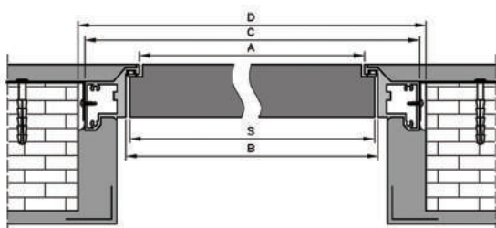
PRZEKRÓJ DRZWI PRZYLGOWYCH
