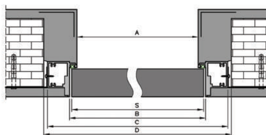
PRZEKRÓJ DRZWI BEZPRZYLGOWYCH
